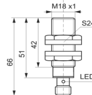
wyjście konektorowe / plug output
