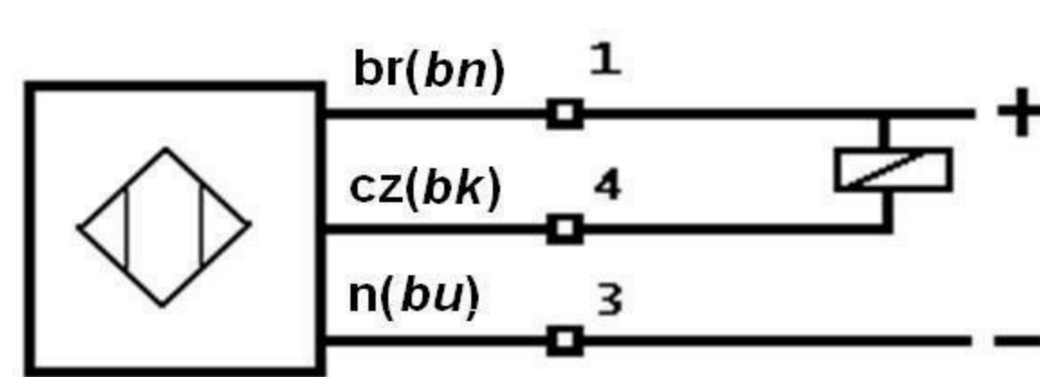
NPN
