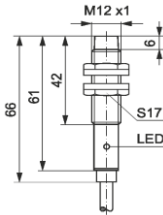
wyjście kablowe / cable output
