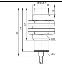
wyjście kablowe / cable output
